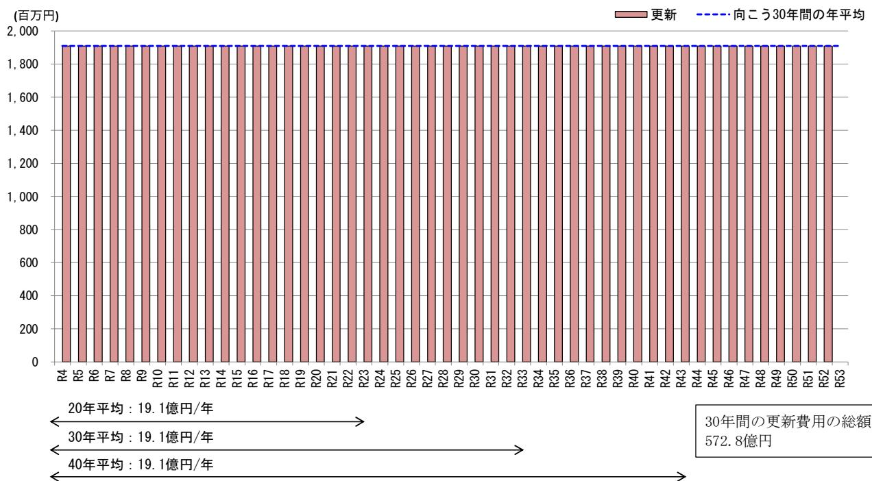
図2-26 下水道（公共下水道・農業集落排水）の将来の更新費用（自然体）の推計
