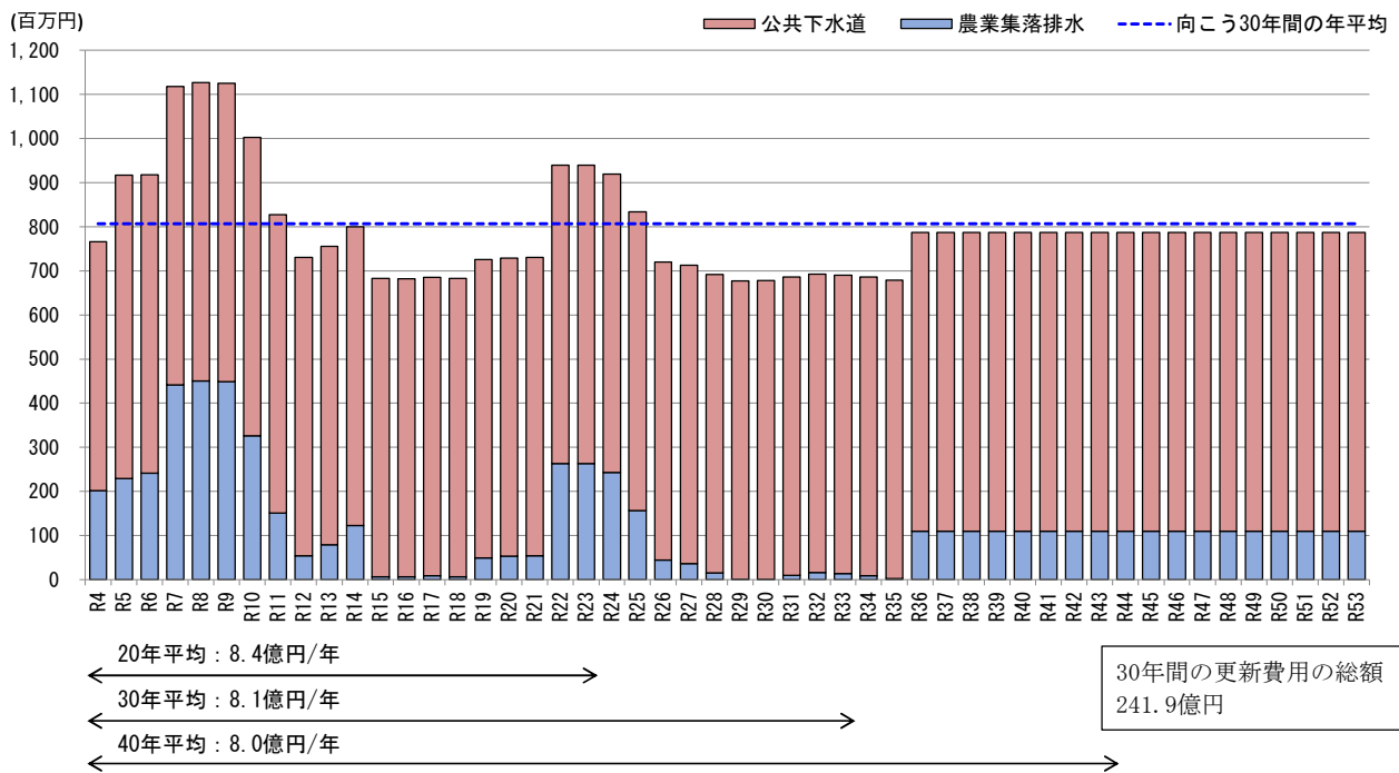
図 2-3 1 下水道（公共下水道・農業集落排水）の将来の更新費用（対策後）の推計
