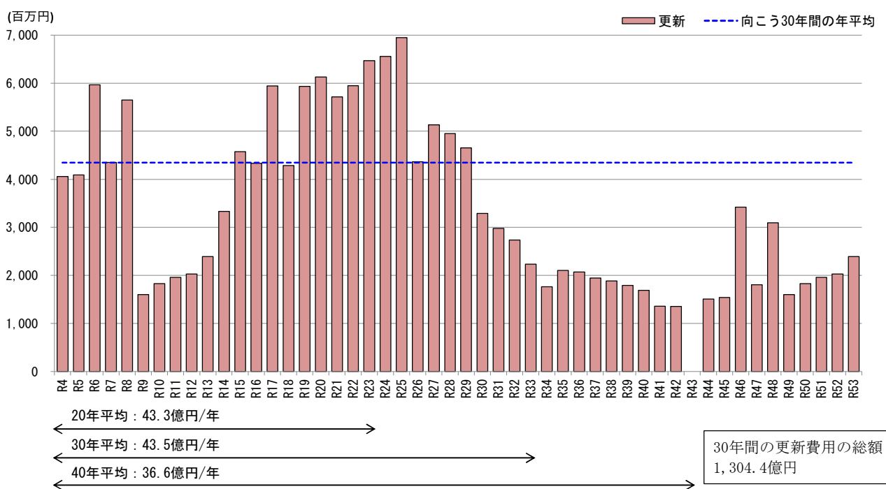
図 2 - 2 5 上水道の将来の更新費用（自然体）の推計
