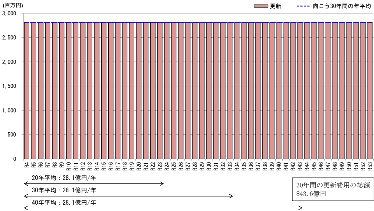
図2-23 道路の将来の更新費用（自然体）の推計
