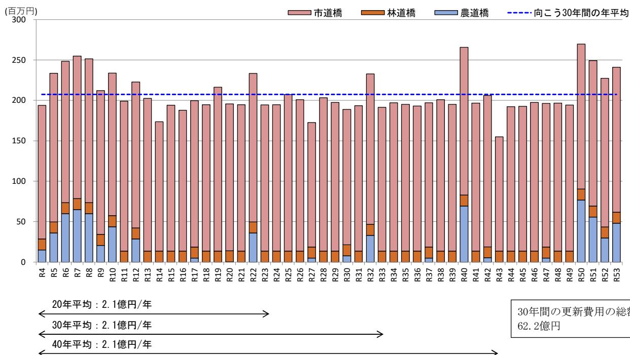
図 2-29 橋りょうの将来の更新費用（対策後）の推計
